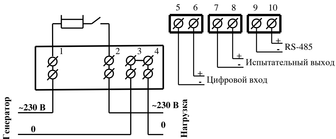
Рисунок А.1 – Схема подключения силовых и интерфейсных цепей счётчиков внутренней установки (СЭБ-1ТМ.03Т – СЭБ-1ТМ.03Т.31)
