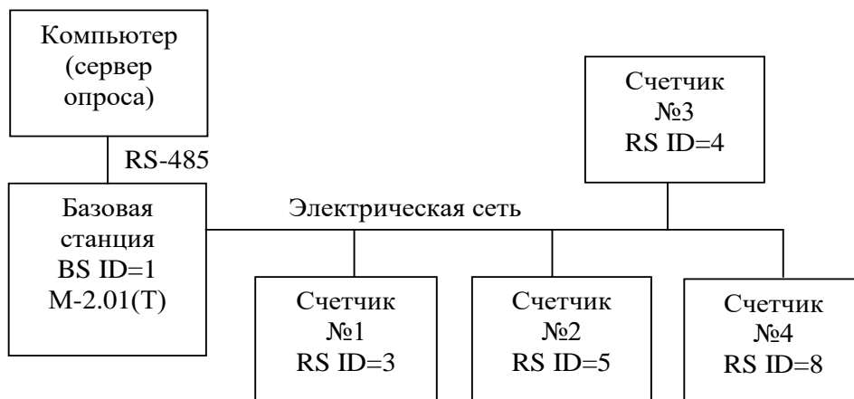
Рисунок 43 – Структурная схема сети передачи данных
