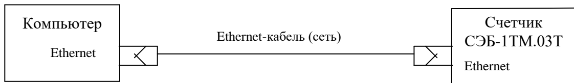
Рисунок Б.7 - Схема подключения счётчика к компьютеру через Ethernet-модем
