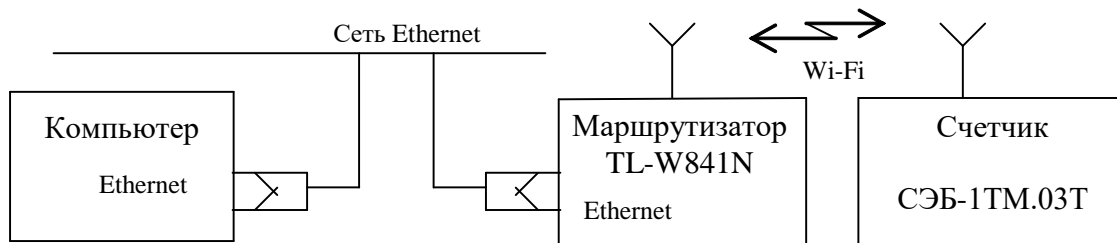
Рисунок Б.6 - Схема подключения счётчика к компьютеру через Wi-Fi-коммуникатор
