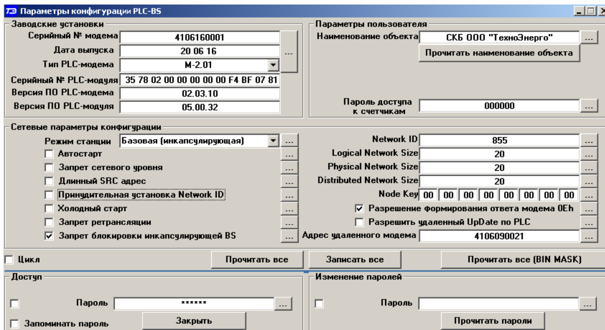
Рисунок 46 – Форма «Параметры конфигурации PLC-модема»
