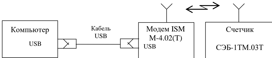
Рисунок Б.5 - Схема подключения счётчика к компьютеру через модем ISM М-4.02(Т)
