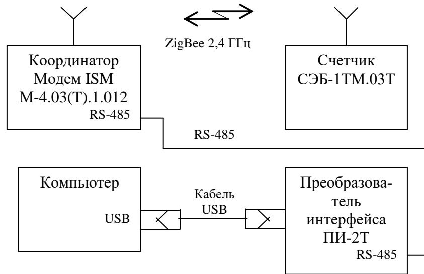
Рисунок Б.8 - Схема подключения счётчика с ZigBee-модемом к компьютеру через координатор М-4.03(Т).1.012
