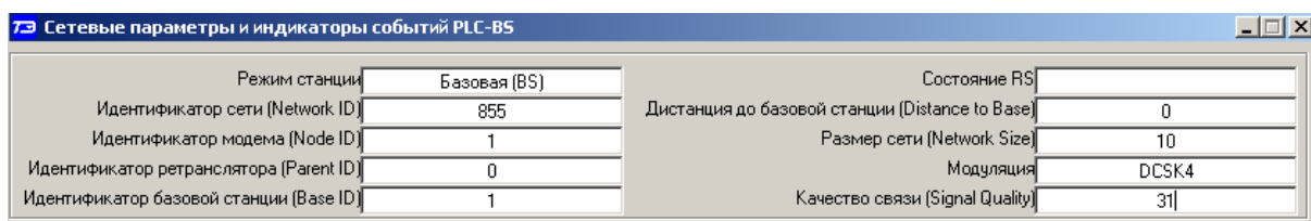
Рисунок 47 – Сетевые параметры PLC-модема M-2.01 в режиме базовой станции
